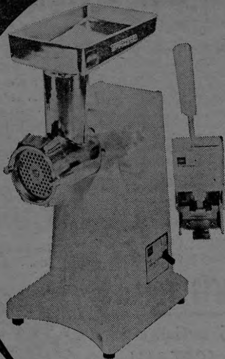
MOLEDORA MT-300 Hace por sí sola muchas cosas: muele carnes, vegetales, frutas, quesos, pescado y nueces. Dos placas cortadoras para cortar fino y grueso. Abre todo tipo de latas y las mantiene puestas hasta que usted las quite. Aditamento para triturar hielo, con lo cual usted puede preparar deliciosos refrescos fríos. Tiene más usos de acuerdo con su propia iniciativa.
